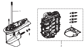
Fig. 23 ASSEMBLY · KIT PARTS アセンブリ・キットパーツ
